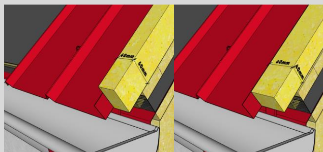
ZALOŽENÍ PRVNÍ ŘADY PŘESAHEM KRYTINY DO ŽLABU
