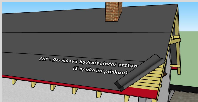
APLIKACE POJISTNÉ HYDROIZOLAČNÍ VRSTVY (DHV)
