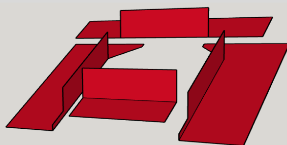
OPLECHOVÁNÍ KOMÍNA, JEDNOTLIVÉ DÍLCE
