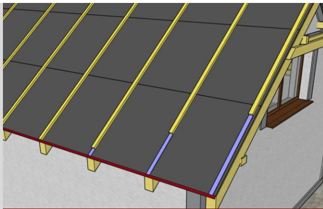
MONTÁŽ KONTRALATÍ
