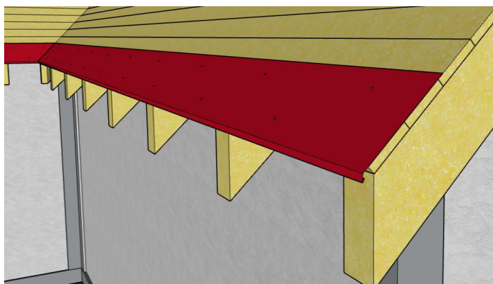
ZALOŽENÍ OKAPNICE POD FÓLIÍ
