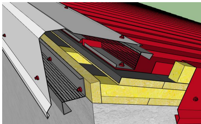
ZAKONČENÍ PULTOVÉ STŘECHY
