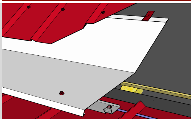
PŘECHOD DO PŮLTOVÉ STŘEŠNÍ ROVINY
