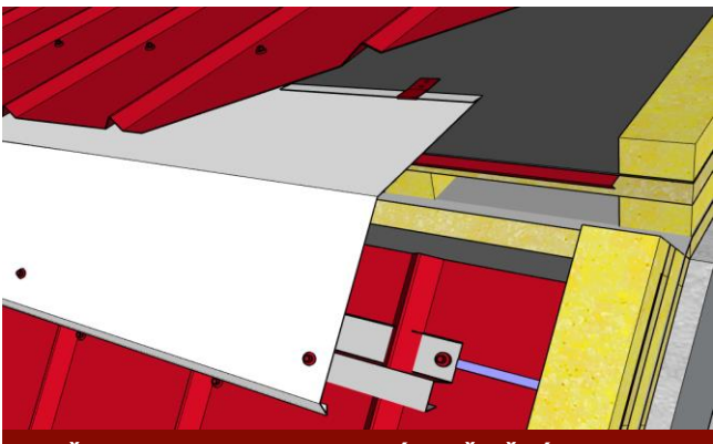
PŘECHOD MANSARDOVÉ STŘEŠNÍ ROVINY
