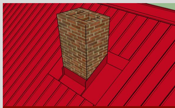
OPLECHOVÁNÍ KOMÍNA – DETAIL
